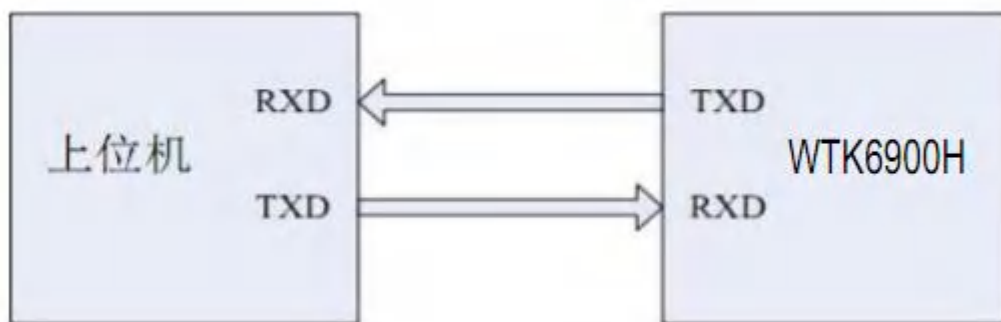
图表 WTK6900HA-16S 芯片 UART 接口连接示意图
